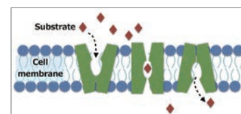
Fig. 2 Membrane transporter
